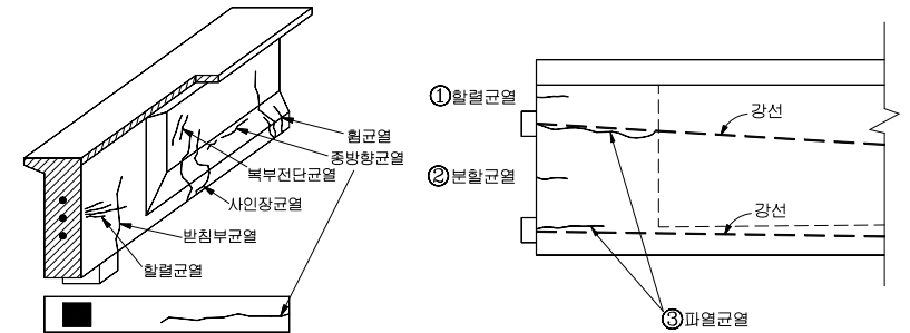
< PSC I빔의 점검부위 >
