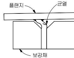
< 피로균열이 발생하기 쉬운 구조상세 >
