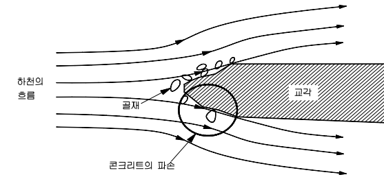
< 유수에 의한 콘크리트 교각의 침식 >
