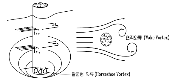
< 수축세굴과 국부세굴 >
