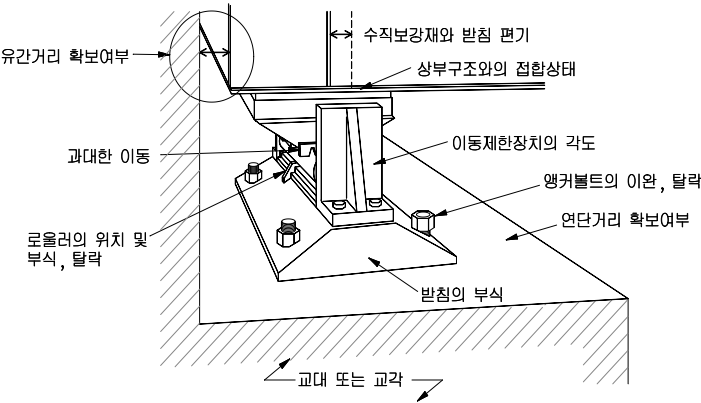
< 교량받침 점검부위 >
