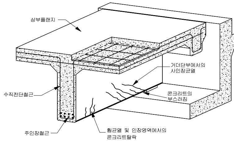
< 철근콘크리트 거더의 점검부위 >
