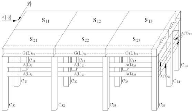
[그림 1.2] 라멘교의 부재 구성도
