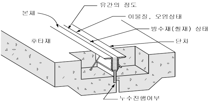
< 신축이음 점검부위 >
