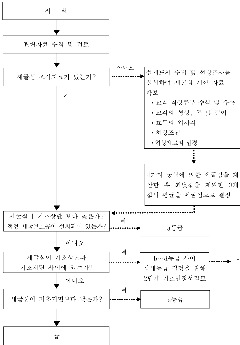
[그림 1.3] 1단계 세굴심 평가 결과 산정 방법
