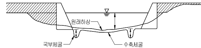
< 수축세굴과 국부세굴 >
