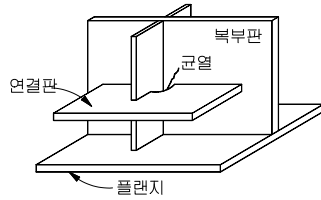
< 피로균열이 발생하기 쉬운 구조상세 >
