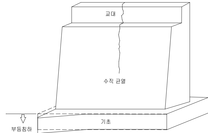
< 부등침하로 인한 교대의 수직균열 >
