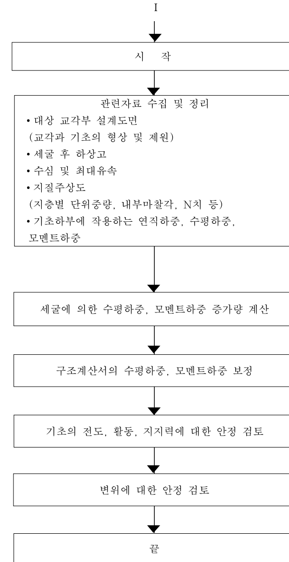
[그림 1.4] 2단계 기초안전성 평가 결과 산정 방법
