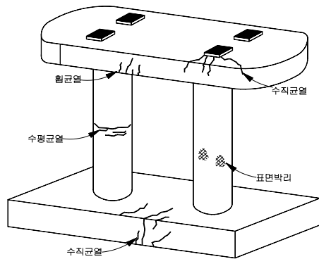
< 콘크리트 교각의 점검부위 >
