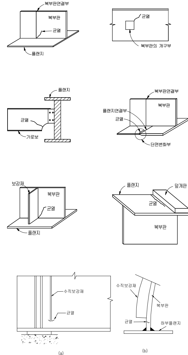
< 피로균열이 발생하기 쉬운 구조상세 >
