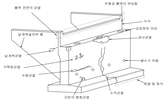
< 교대의 점검부위 >
