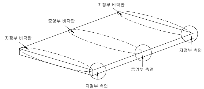
< 거더가 없는 경우의 바닥판 점검부위 >
