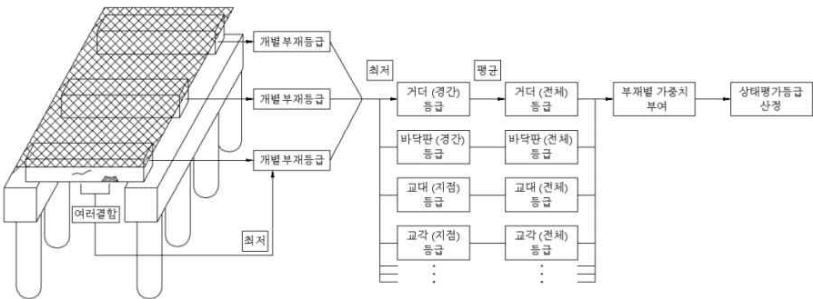
[그림 1.1] 전체 교량의 상태평가결과 산정 방법 예
