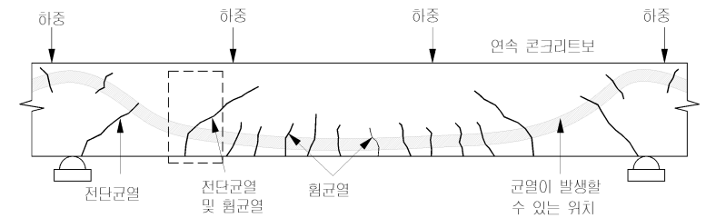
< 콘크리트 거더에 발생하는 균열의 유형과 위치 >
